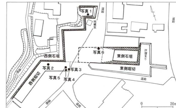
富岡城 新大手門平面図
