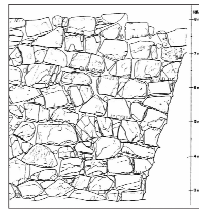
図1 石垣の図化
