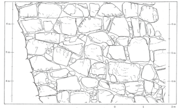
図1 石垣Cの修復前の図面(写真1の部分)
