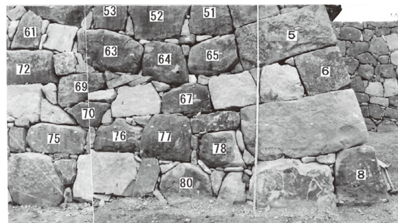
写真2 石垣A(東側)修復後(標高5.5~3m部分)
