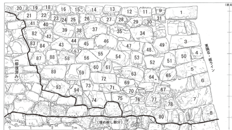
図1 石垣A(東側)修復前
