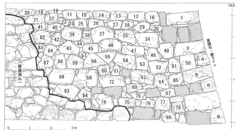
図2 石垣A(東側)修復後 ※スクリーントーンは新しい石
