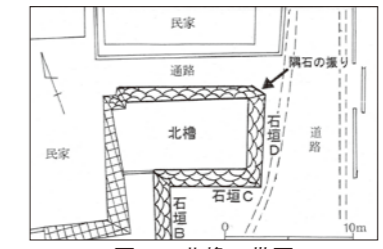
図3 北櫓一帯図
