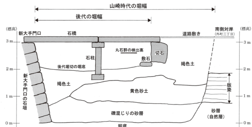
図1 新大手門・堀切 イメージを加えた断面図
