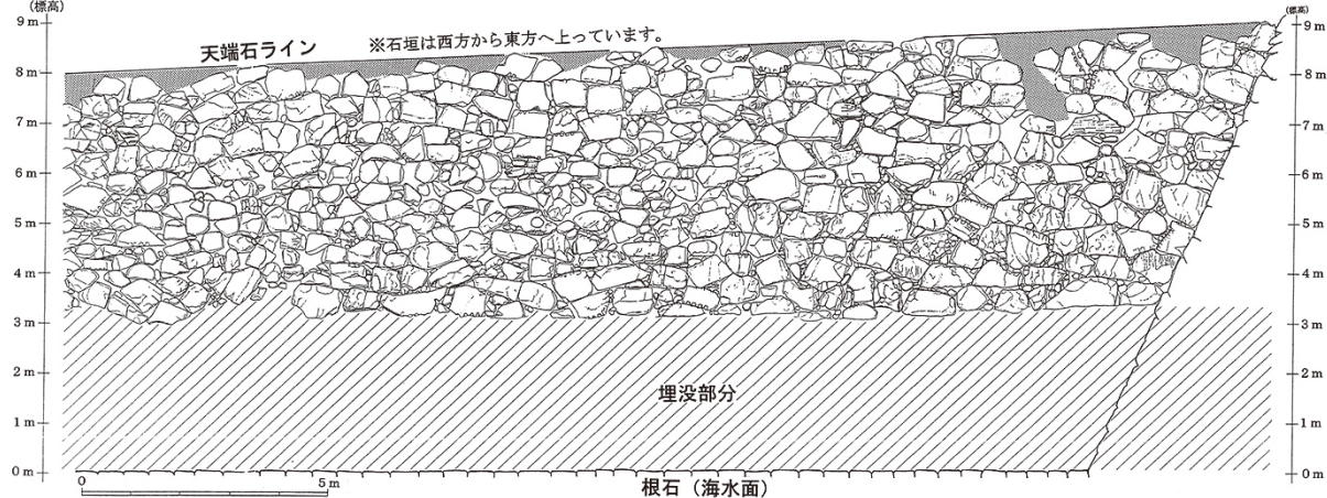
図2 百間石垣実測図（東端部より22m分）※長堀の復元工事に伴う調査
