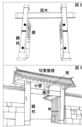
図2 冠木門 図3 高麗門
