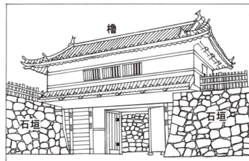
図1 櫓門 〔甲府城 山手渡櫓門 背面のスケッチ〕 (所在地: 山梨県甲府市)
