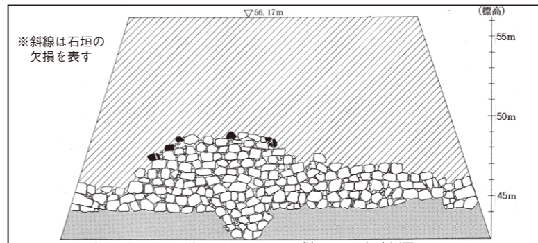
西側4面 石垣実測図
