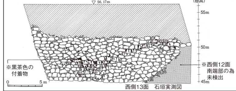
西側13面 石垣実測図
