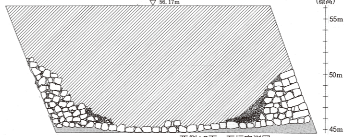
西側12面 石垣実測図
