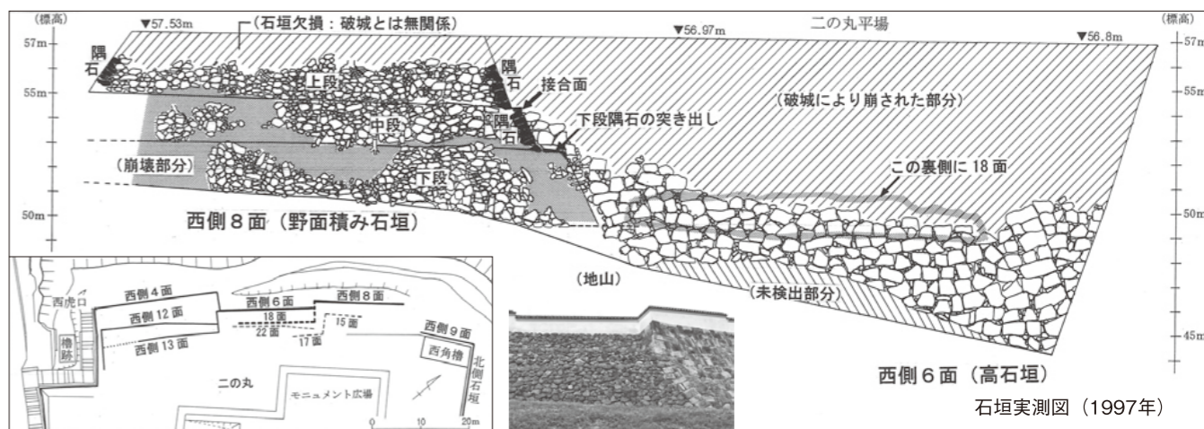
二の丸平面図(西側)と高石垣の検出状況
